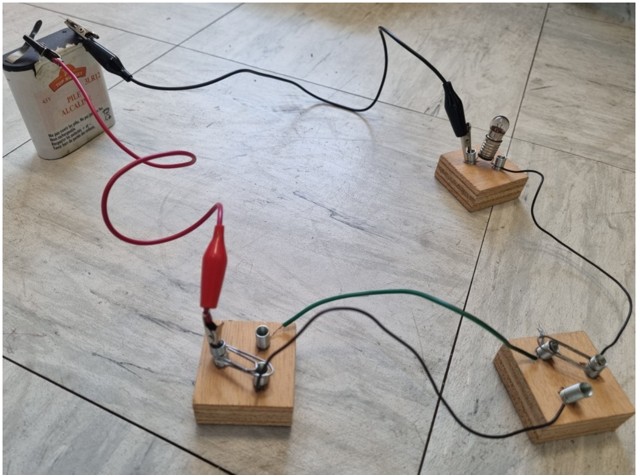
Exemple de montage « Circuit Va-et-vient »
